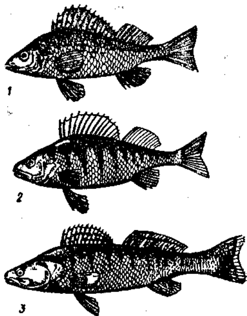
Рис. 36. Родина окуневих:
